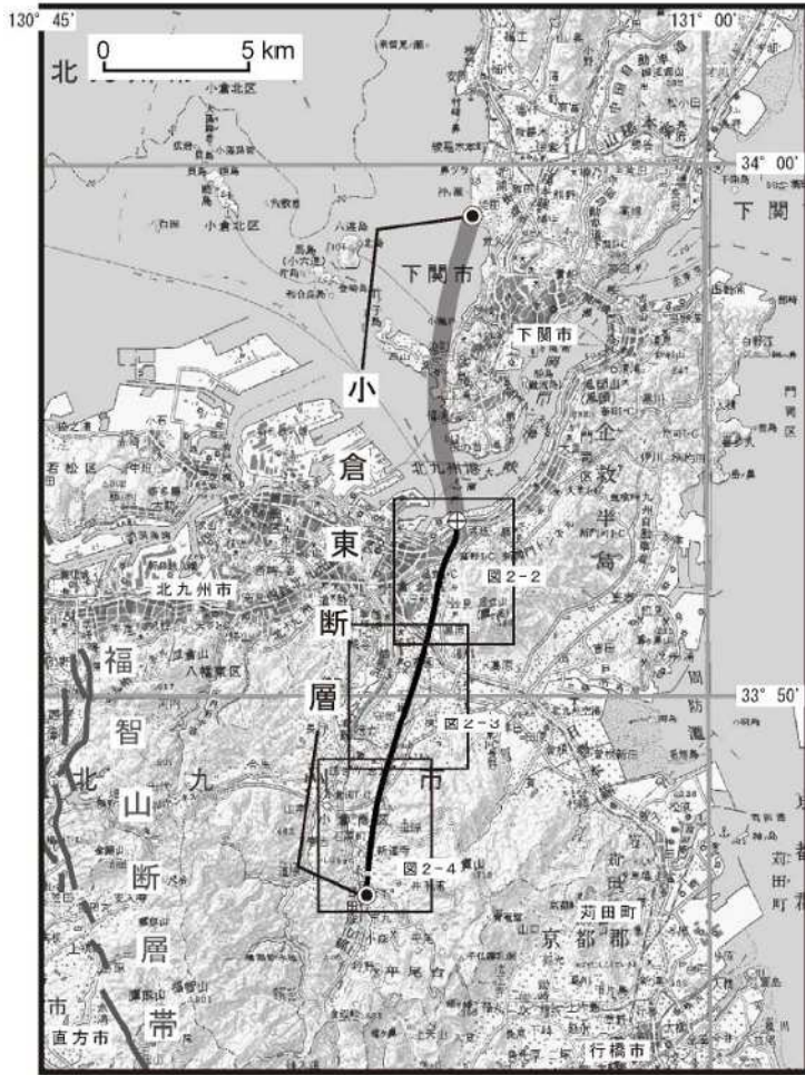
図 小倉東断層位置 (地震調査研究本部ホームページ参照 http://jishin.go.jp/main/chousa/13feb_chi_kyushu/k_1.pdf )
